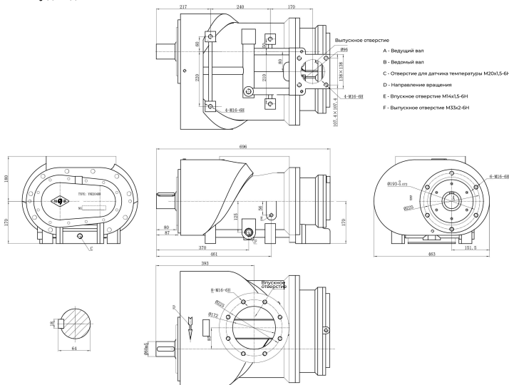
Общий вид компрессорного блока YNE204RB
