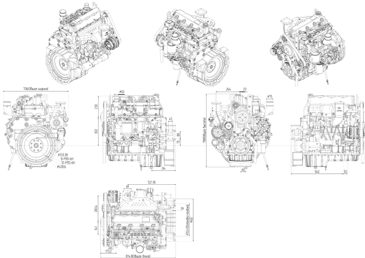
Схема двигателя DEF47CDT4
