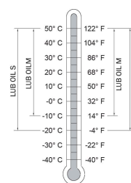
Масло компрессора
