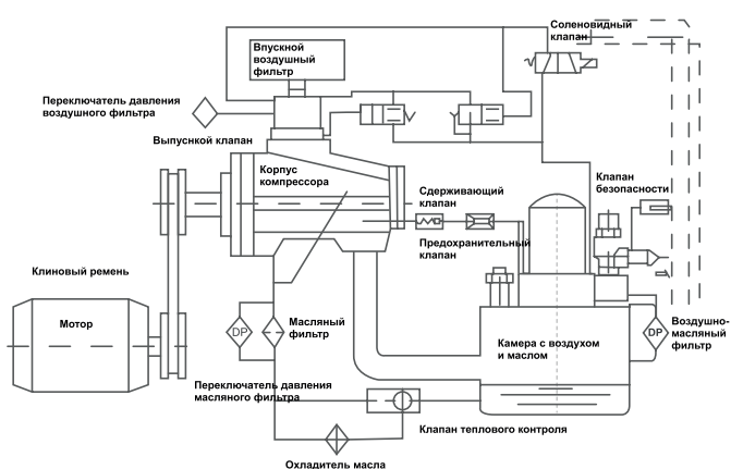
Схема технологического процесса (22 кВт и ниже)
